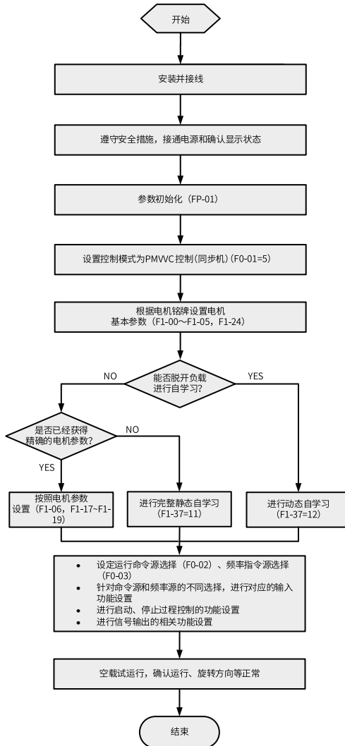
图2-4 变频器调试流程图 (PMVVC控制)
