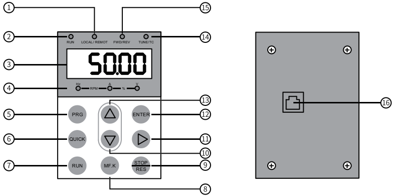
图1-2 部件示意图
